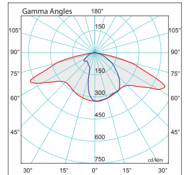
Işık Şiddeti Dağılımı Eğrisi Light Distribution Curve
