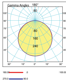
Işık Şiddeti Dağılım Eğrisi Light Distribution Curve
