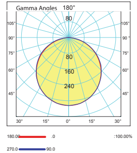
Işık Şiddeti Dağılım Eğrisi Light Distribution Curve
