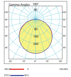
İşık Şiddeti Dağılım Eğrisi Light Distribution Curve
