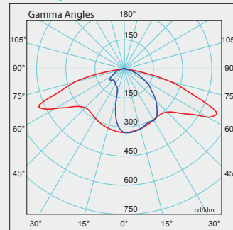
Işık Şiddeti Dağılım Eğrisi Light Distribution Curve
