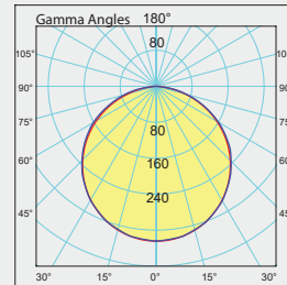
Işık Şiddeti Dağılım Eğrisi Light Distribution Curve
